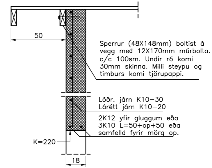
Festiplata í innvegg 1:10
