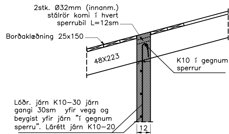
Sérmynd 13 1:20 1702
