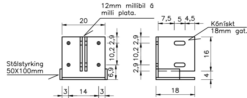
Festiplata í útvegg 1:10
