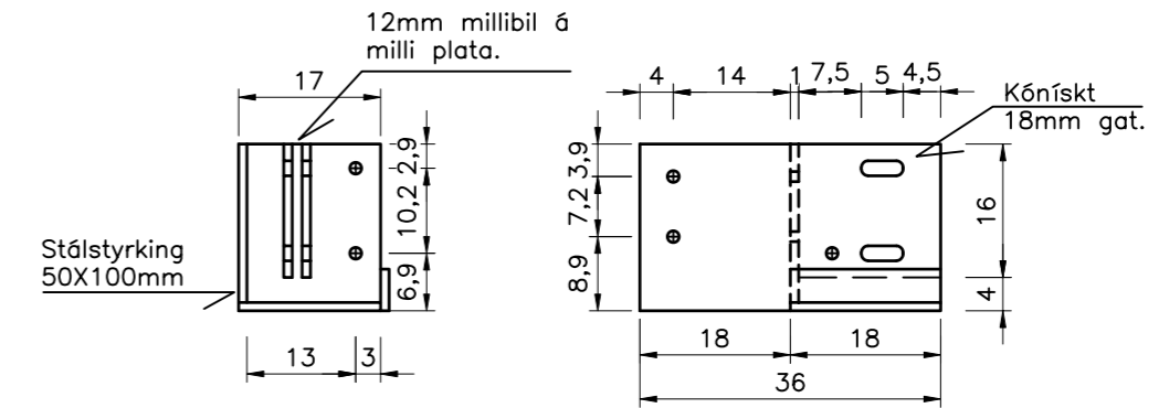
Festiplata í innvegg 1:10
