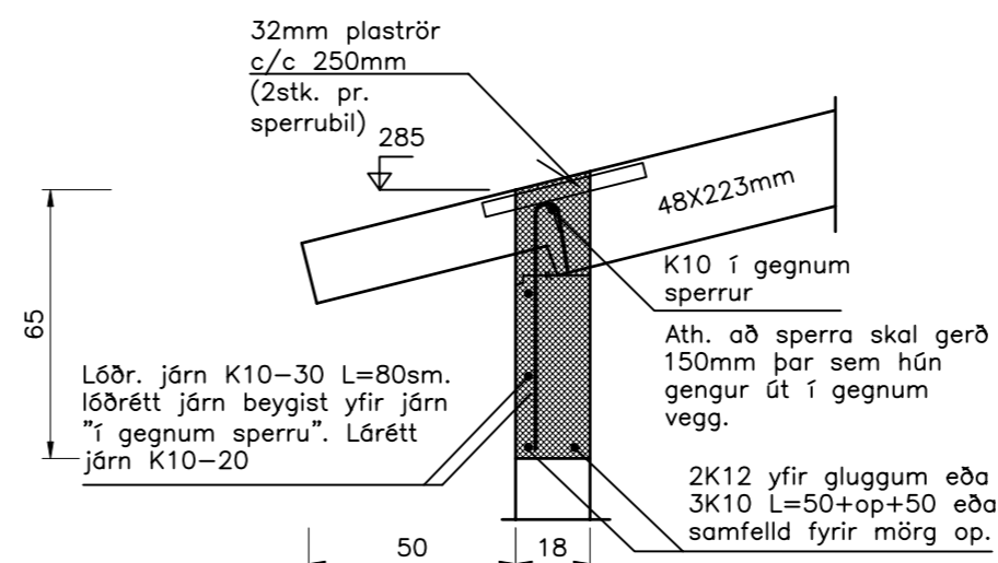
Snið 6 1:20 1702
