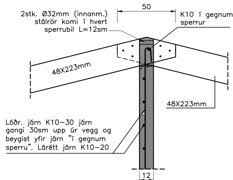
Snið 16 1:20 1702
