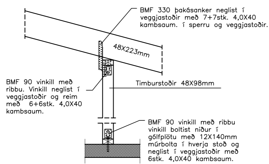
Sérmynd 14 1:20 1702
