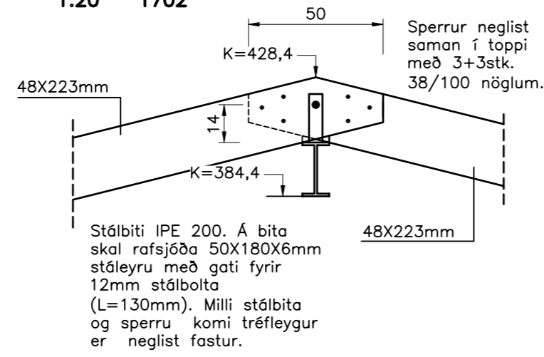
Snið 12 1:20 1702
