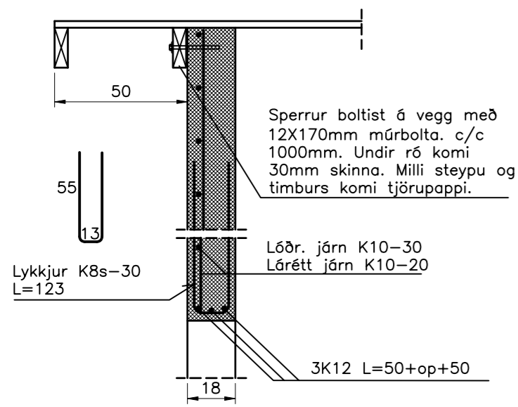
Snið 11 1:20 1702
