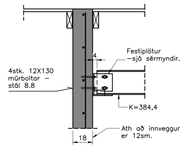
Sérmynd 9 1:20 1702
