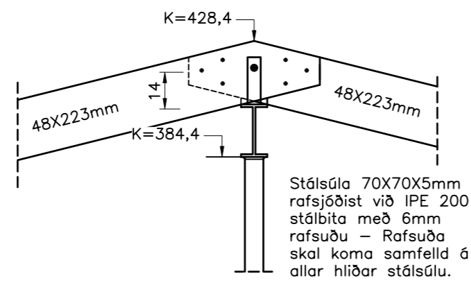
Snið 12 1:20 1702
