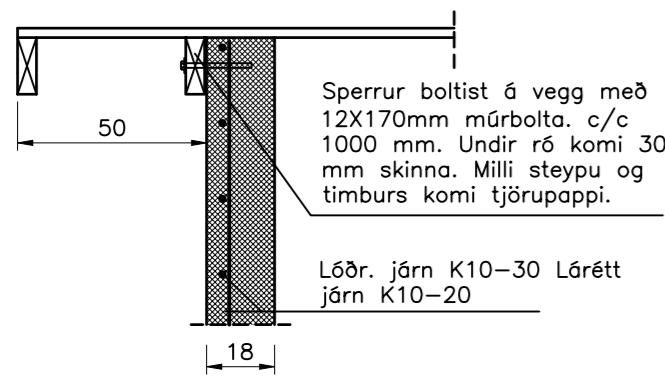
Snið 11 1:20 1702
