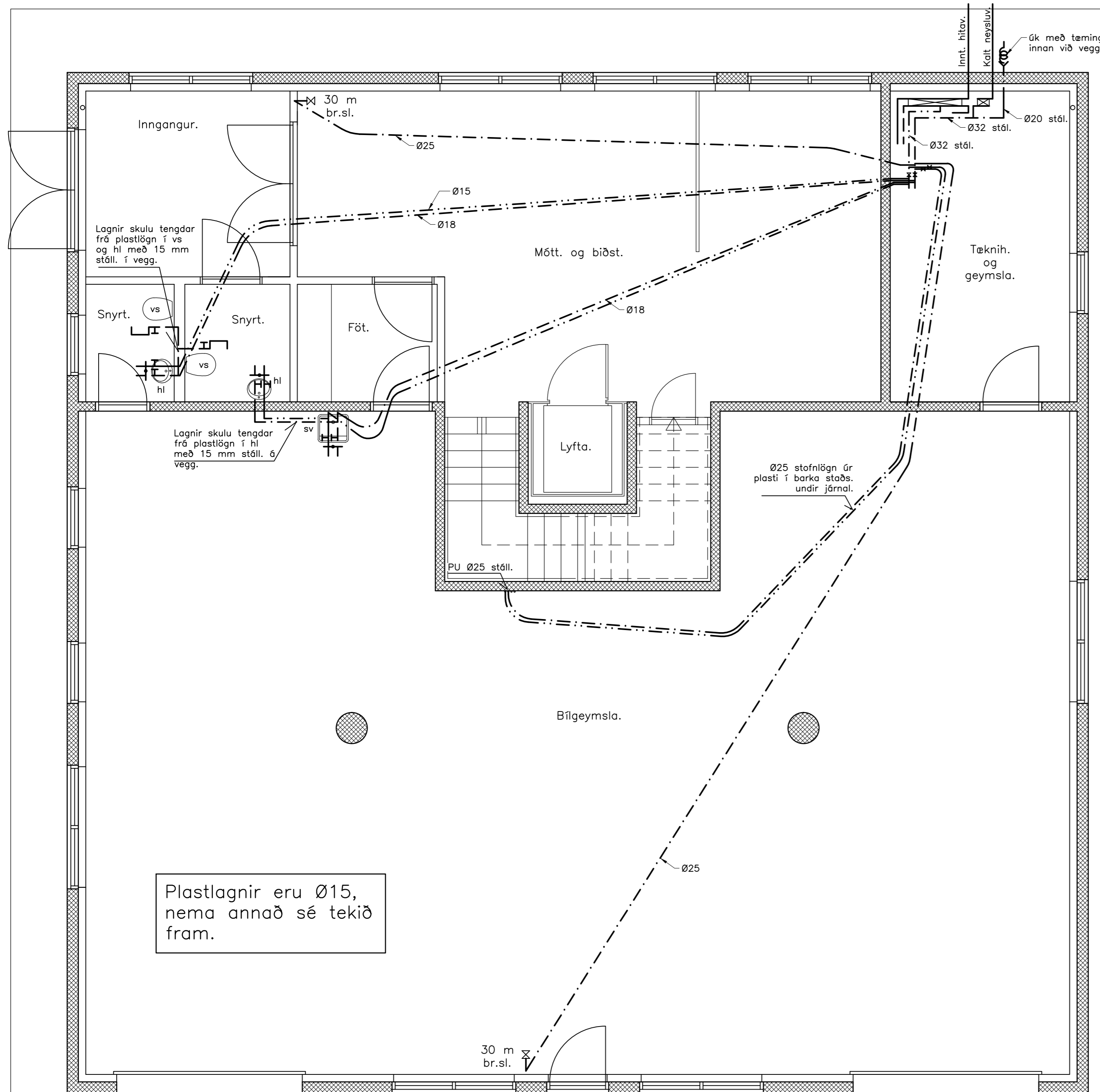
Grunnmynd 1.hæðar 1:50
