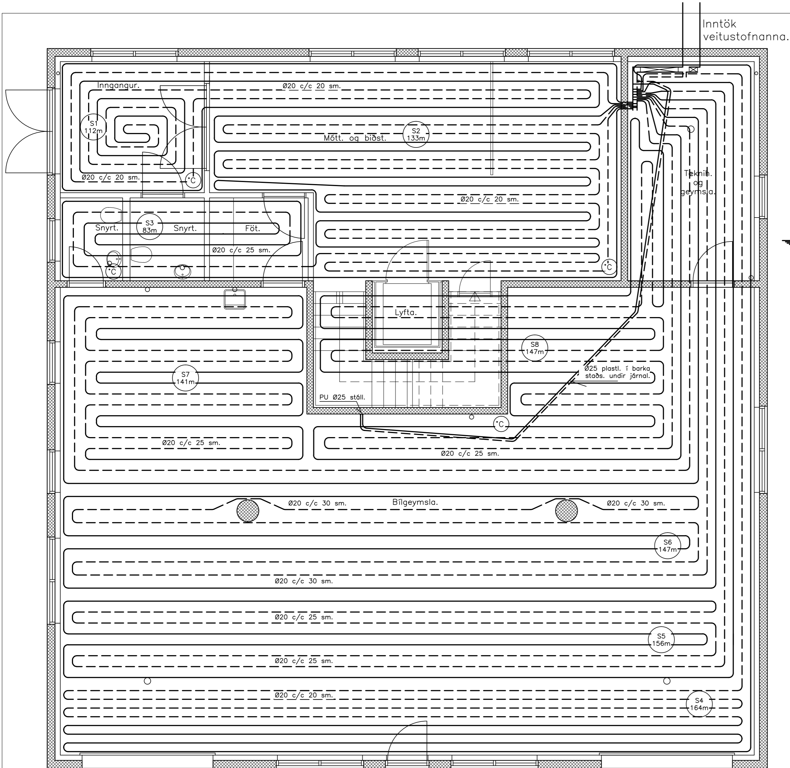
Grunnmynd 1.hæðar 1:50
